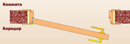
Открывание двери в коридор (петли правые)
