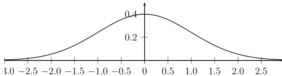
איור 2.2: גרף ההתפלגות הנורמלית הסטנדרטית
