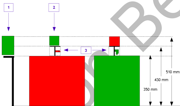
Figure 15 : Schéma de positionnement des balises sur les robots
