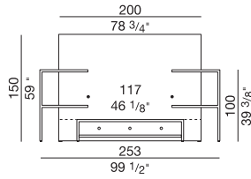
EL 282 prof/depth cm 35/60, h cm150
