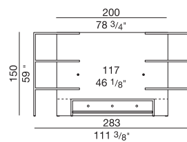
EL 286 prof/depth cm 35/60, h cm150
