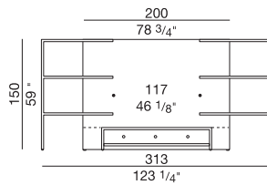
EL 298 prof/depth cm 35/60, h cm150
