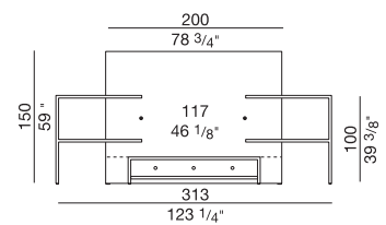
EL 288 prof/depth cm 35/60, h cm150
