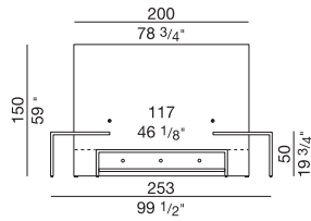
EL 281 prof/depth cm 35/60, h cm150
