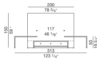
EL 287 prof/depth cm 35/60, h cm150
