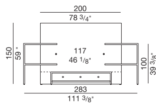
EL 298 prof/depth cm 35/60, h cm150
